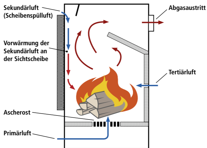
Verbrennungsluftführung im Ofen
